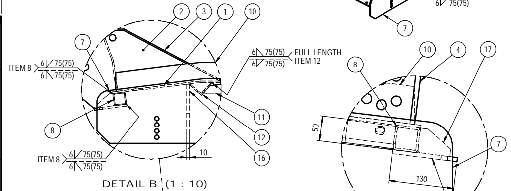
DETAIL B (1 : 10)
