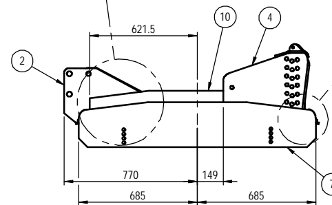
DETAIL B (1 : 10)
