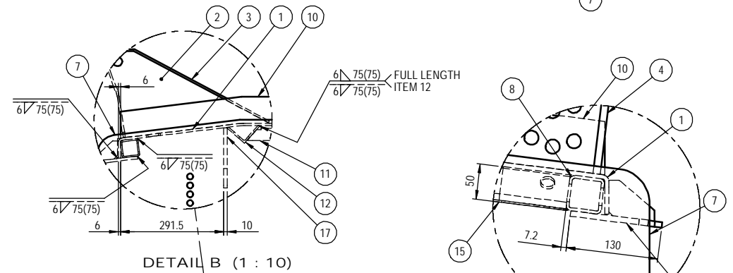
DETAIL B (1 : 10)
